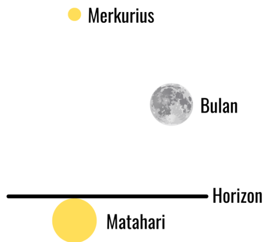
Gambar 11. Ilustrasi posisi Bulan dan Merkurius saat Matahari terbenam
