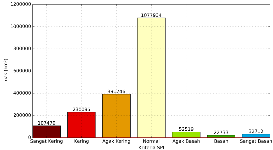
Indeks Presipitasi Terstandarisasi 1 Bulanan Bulan Oktober 2023
