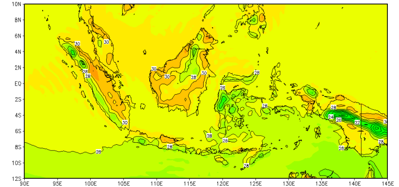
Prediksi Suhu Permukaan Maksimum Dasarian I Juli 2022
