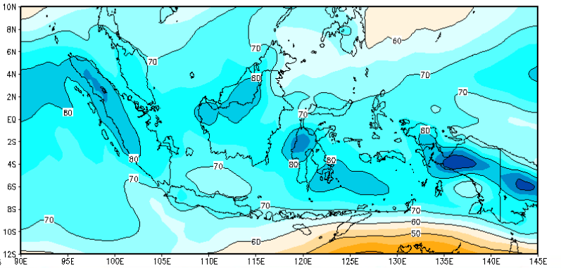
Prakiraan RH 700mb Dasarian I Juli 2022
