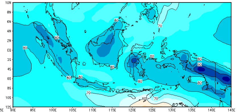
Prakiraan RH 850mb Dasarian I Juli 2022
