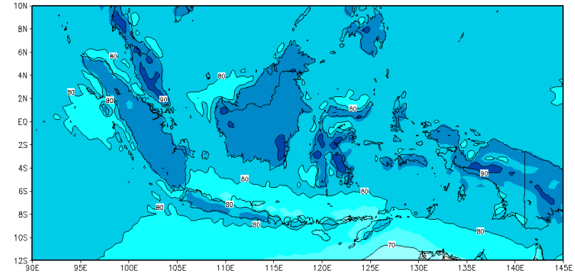
Prediksi RH Permukaan Dasarian I Juli 2022
