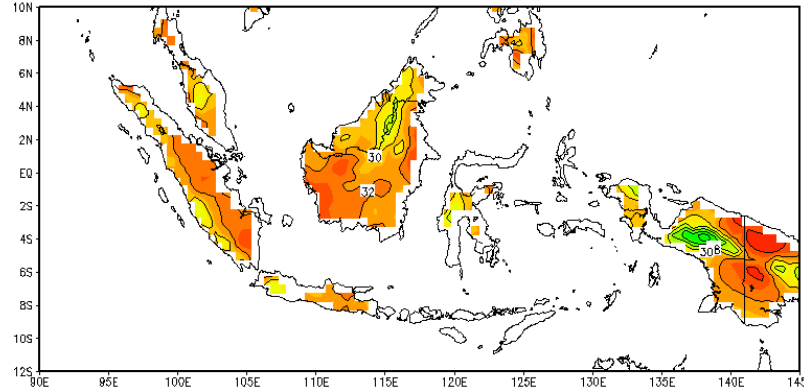
Prediksi Suhu Permukaan Maksimum Dasarian III Juni 2022
