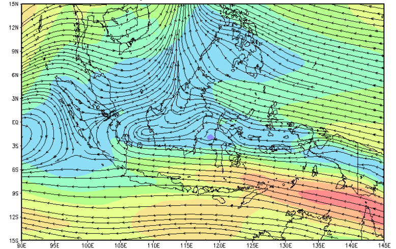
Prediksi Angin 850mb Dasarian II Juni 2022
