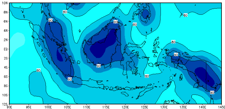
Prediksi RH Permukaan Dasarian III Juli 2022
