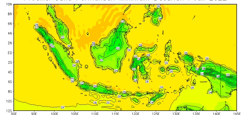
Prediksi Suhu Permukaan Minimum Dasarian I Juli 2022
