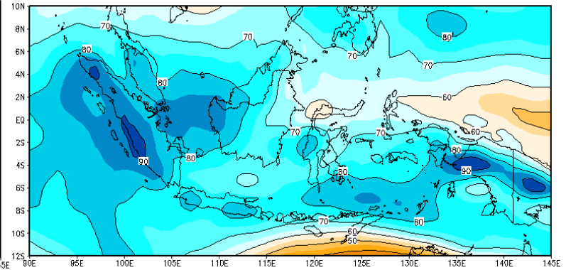
Prakiraan RH 700mb Dasarian I Juli 2022
