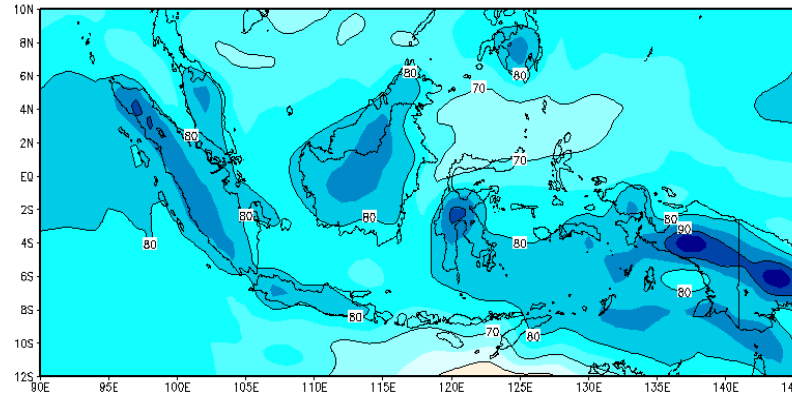
Prakiraan RH 850mb Dasarian III Juni 2022
