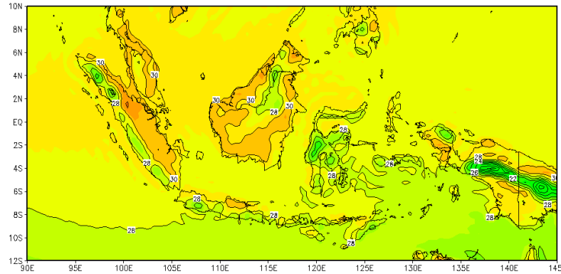
Prediksi Suhu Permukaan Maksimum Dasarian III Juni 2022
