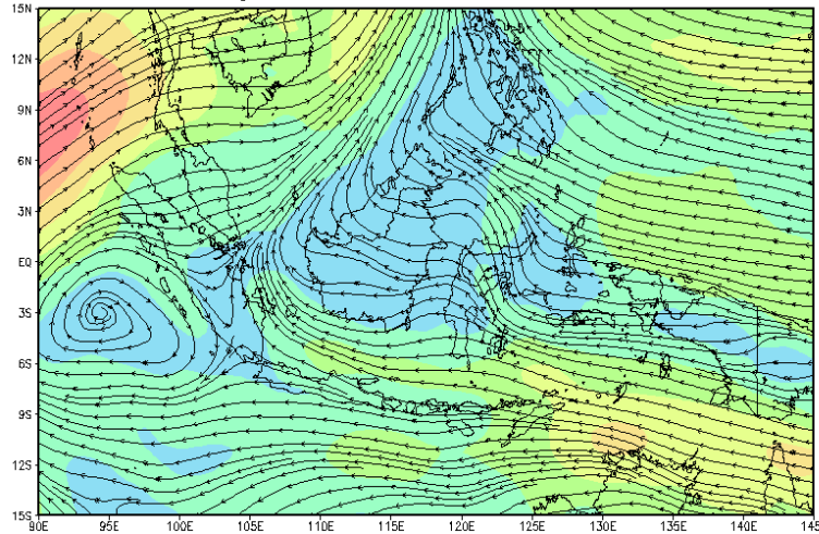
Angin 850mb Dasarian I Juni 2022
