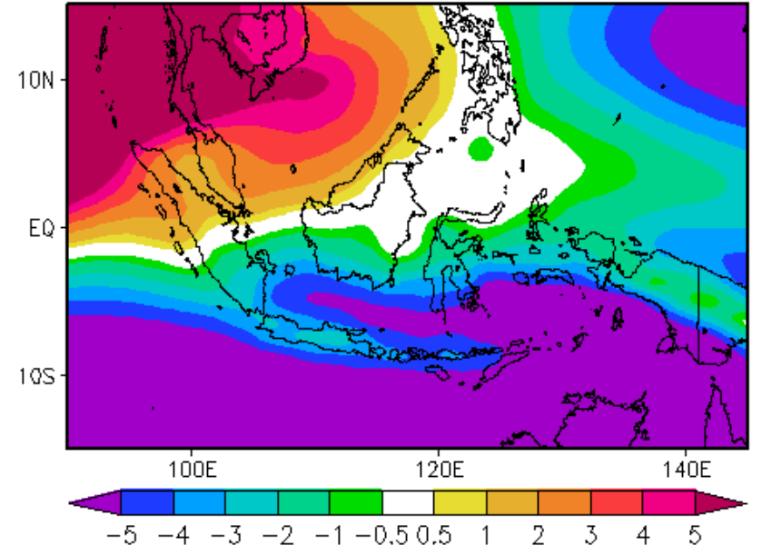
Normal Angin Zonal 850mb Dasarian I Juni
