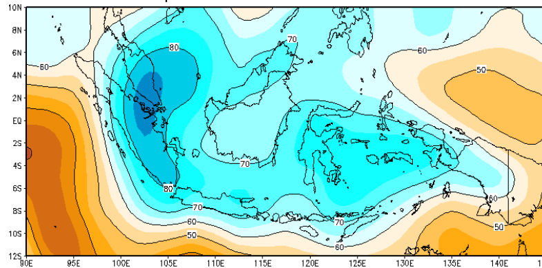
Prakiraan RH 700mb Dasarian III Juni 2022
