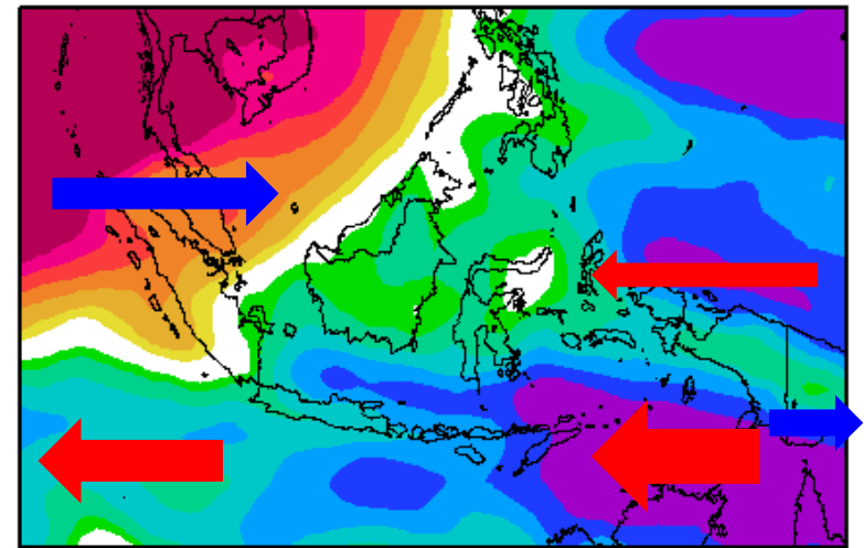
Normal Angin Zonal 850mb Dasarian I Juni
