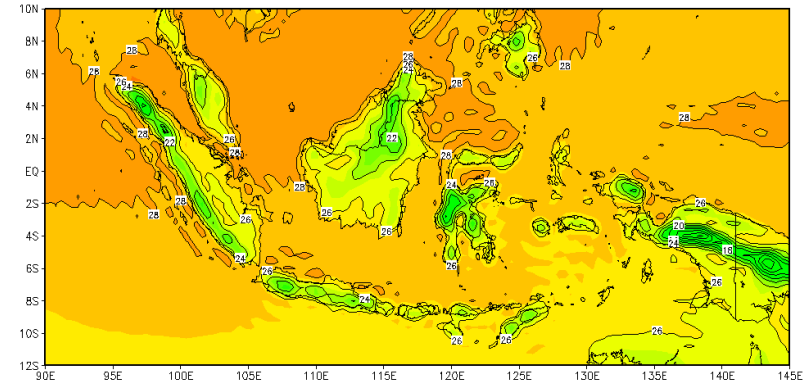
Prediksi Suhu Permukaan Rata-rata Dasarian I Juli 2022
