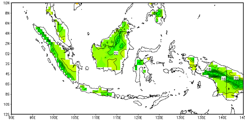
Prediksi Suhu Permukaan Minimum Dasarian III Juni 2022
