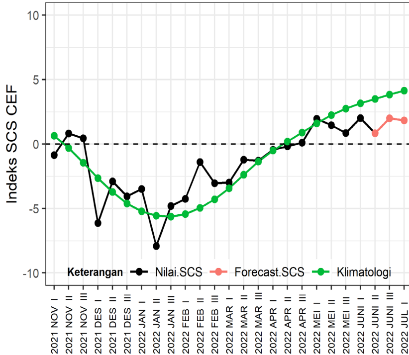
Indeks SCS CEF
