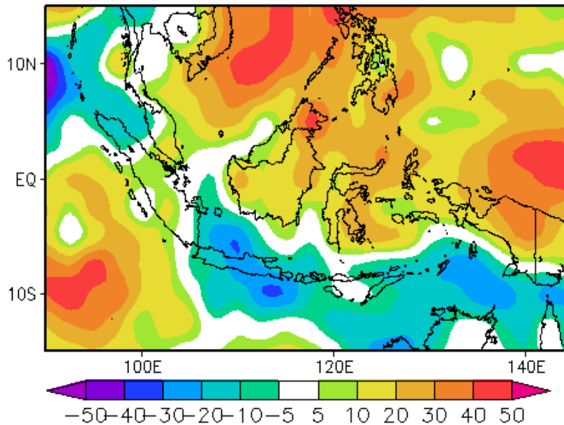
Anomali OLR Dasarian I Juni 2022
