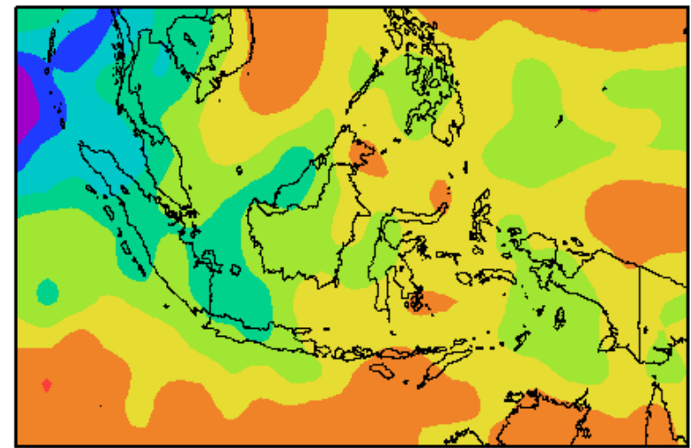
Normal OLR Dasarian I Juni 2022
