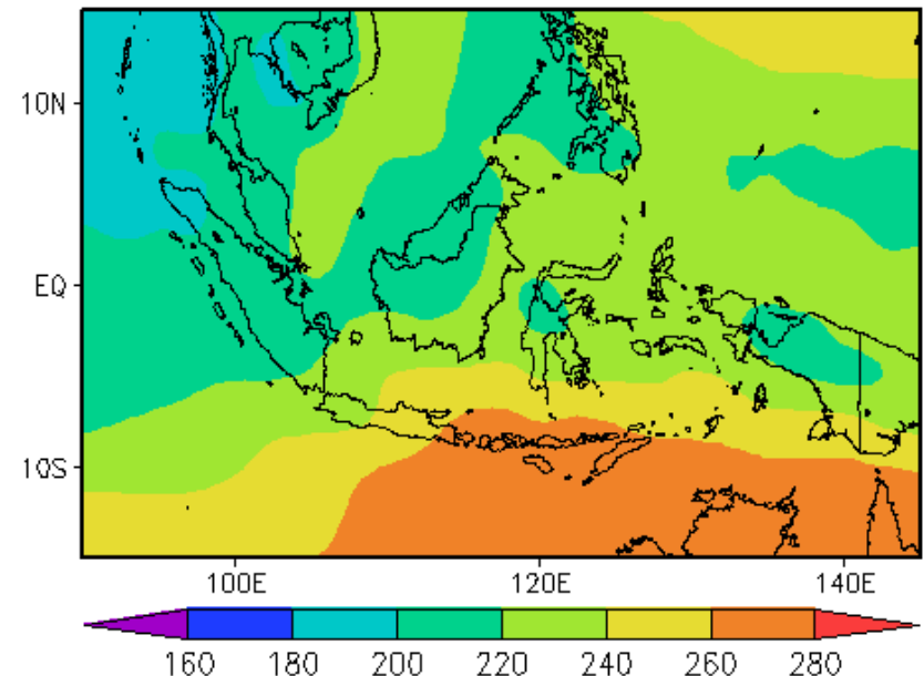
Normal OLR Dasarian I Juni 2022
