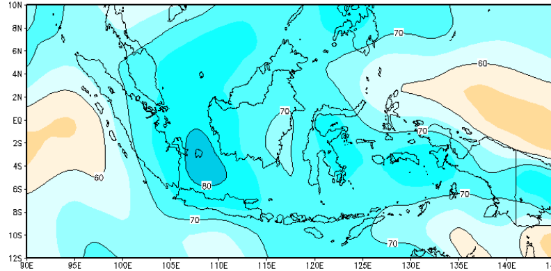
Prakiraan RH 850mb Dasarian III Juni 2022
