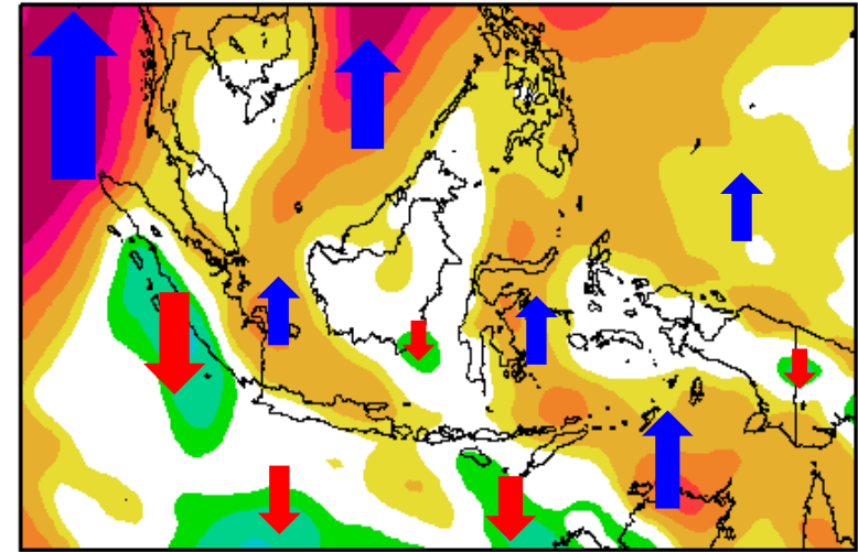
Normal Angin Meridional 850mb Dasarian I Juni
