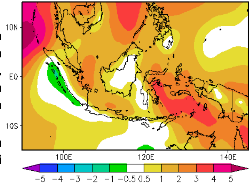
Normal Angin Meridional 850mb Dasarian I Juni
