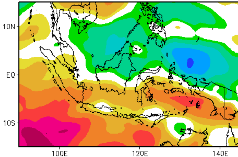
Anomali Angin Zonal 850mb Dasarian I Juni 2022
