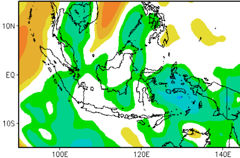
Anomali Angin Meridional 850mb Dasarian I Juni 2022
