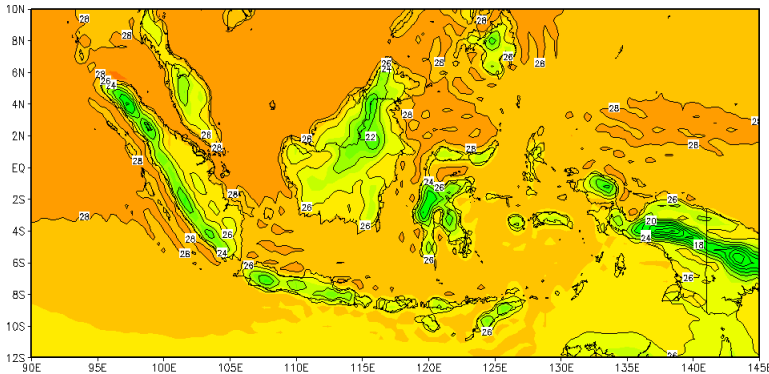
Prediksi Suhu Permukaan Rata-rata Dasarian III Juni 2022
