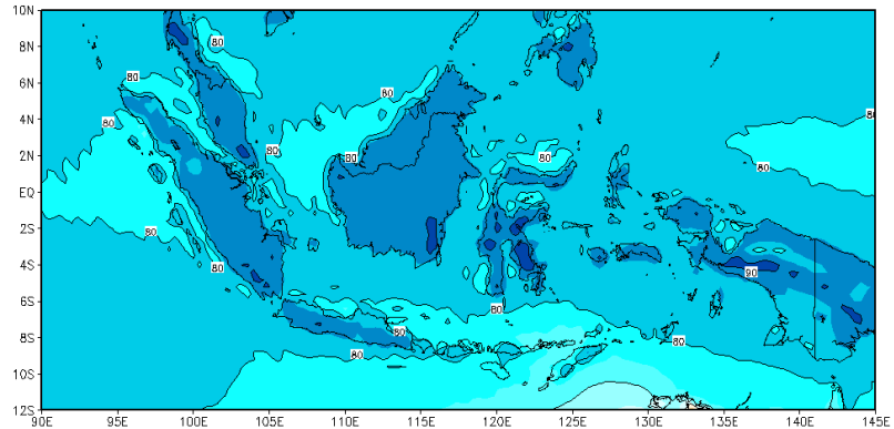
Prediksi RH Permukaan Dasarian I Juli 2022
